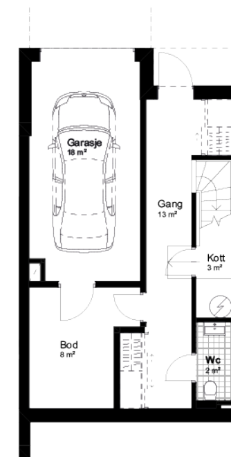
1. ETASJE
