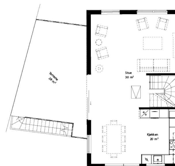
2. ETASJE
