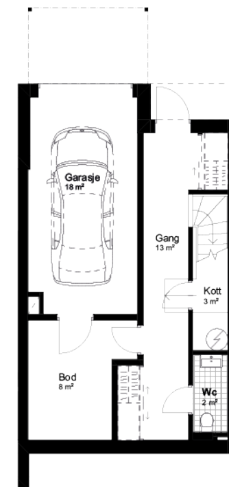
U. ETASJE
