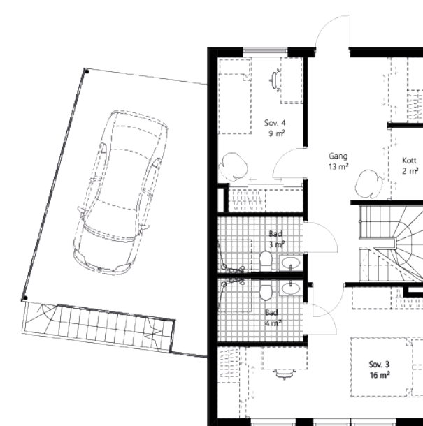
1. ETASJE
