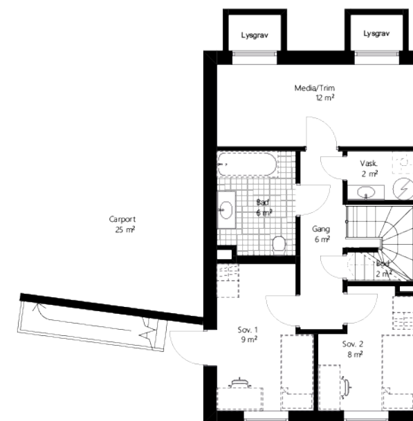
U. ETASJE
