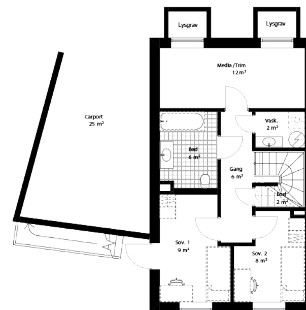
U. ETASJE
