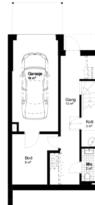
1. ETASJE
