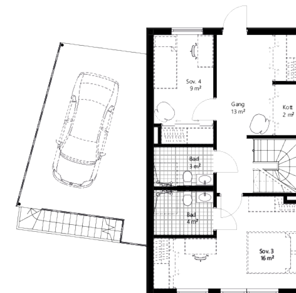
1. ETASJE
