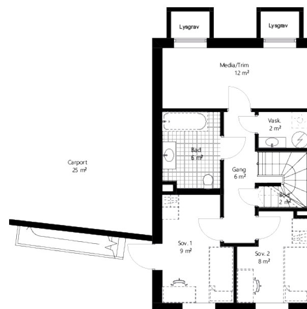
U. ETASJE
