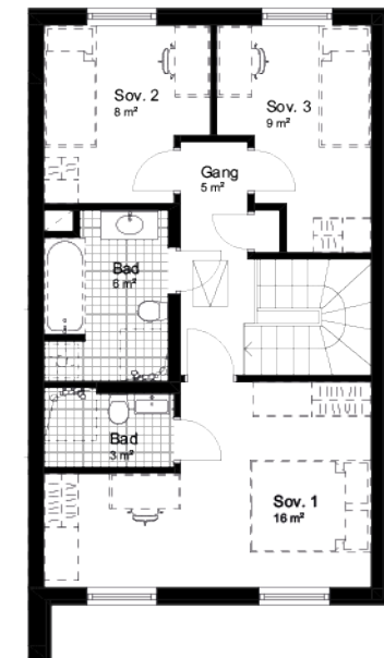
2. ETASJE
